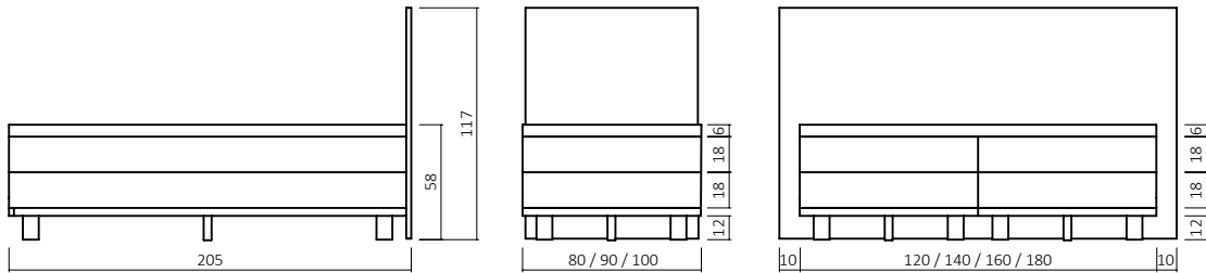
Bsp. Außenmaße (cm) alle Bettgrößen
