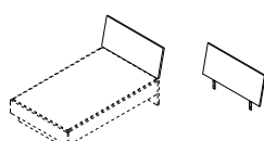
Bettkopfteil in Korpusfarbe mit 12 Grad Halterung, Abstand zur Wand 11,5 cm
