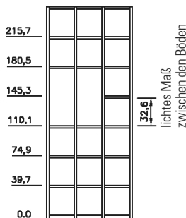
Maßkette bei Wangenhöhen 3, 4, 5, 6, 7 Raster
